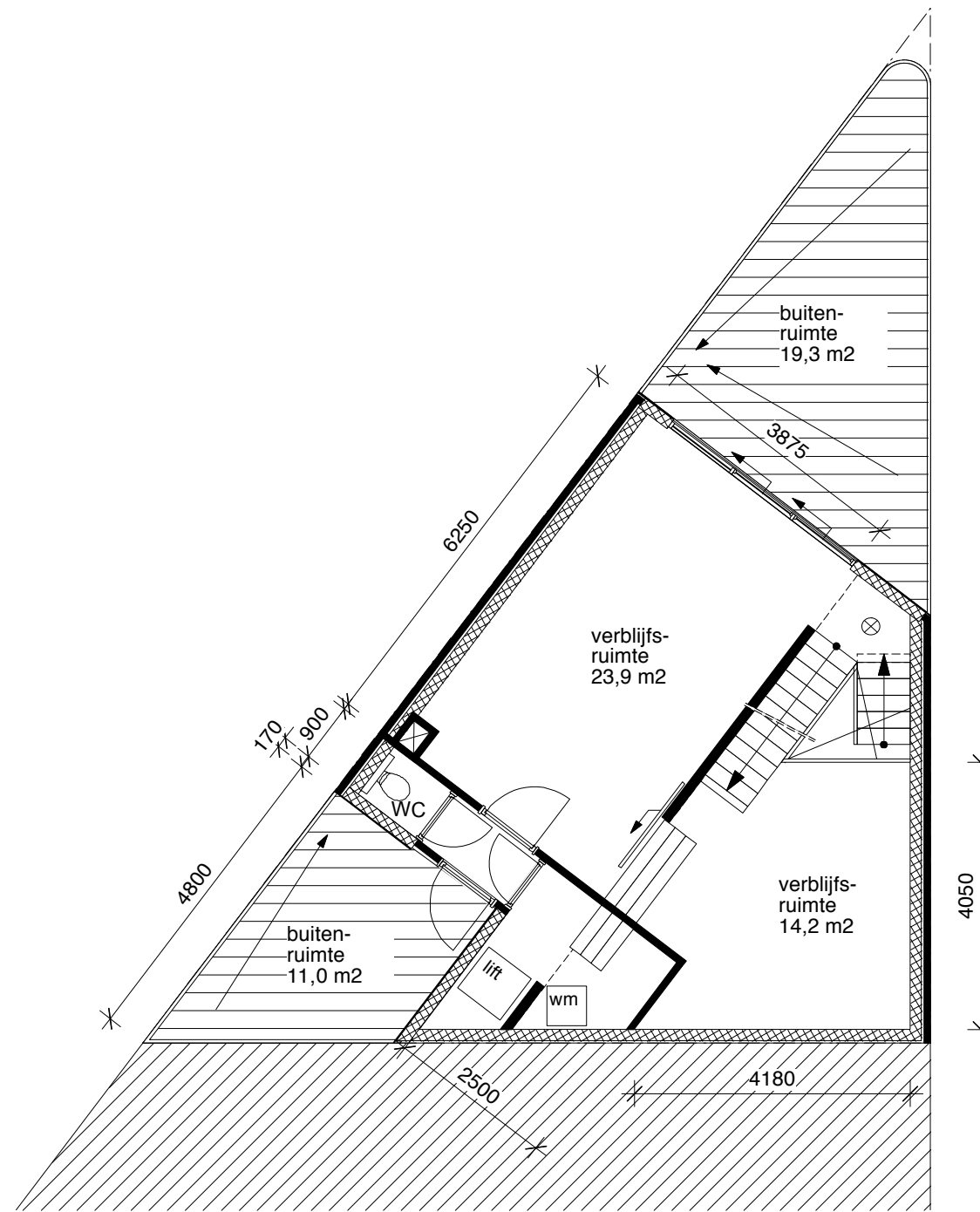
EERSTE VERDIEPING - MULTIFUNCTIONELE RUIMTE - WOONKAMER
