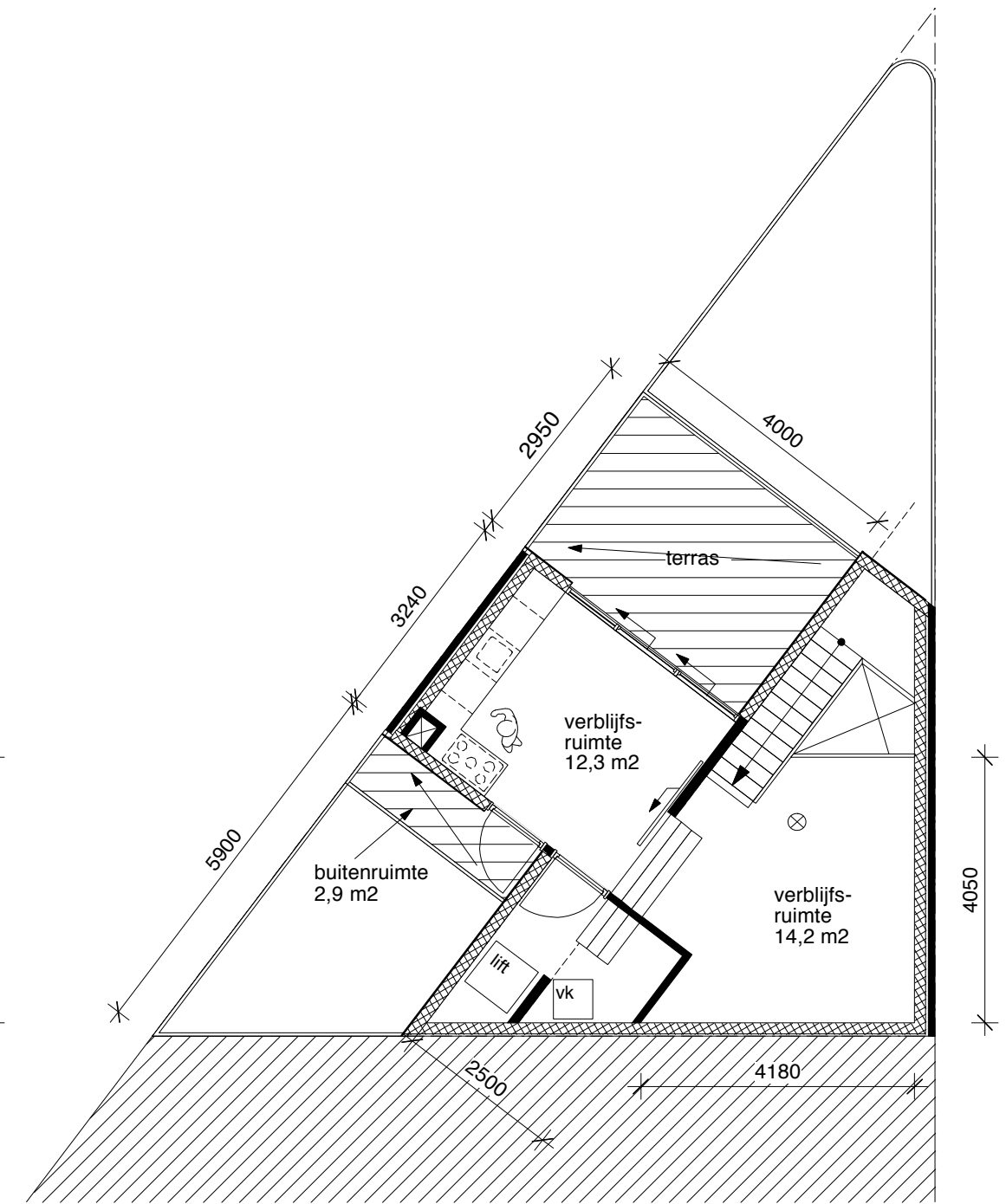
TWEDE VERDIEPING - EETKAMER - KEUKEN
